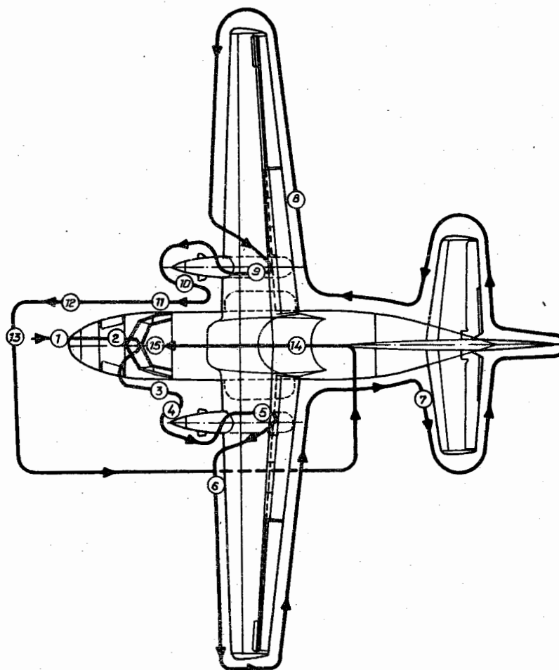
Abb. 4.2.1/1 Übernahmekontrollgang
