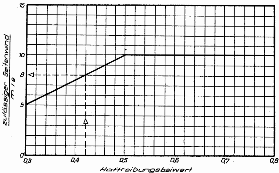
Abb. 2.6.2/1 Haftreibungsbeiwert
