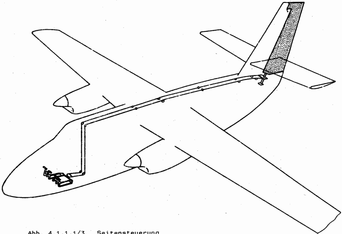
Abb. 4.1.1.1/3 Seitensteuerung
