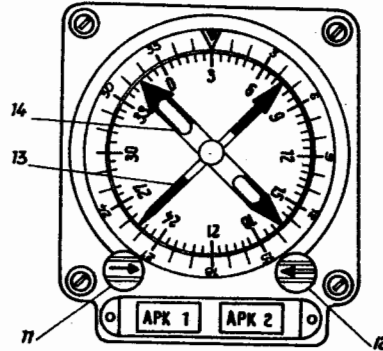
Anzeigegerät IKU-1A
