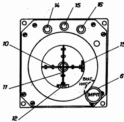
Anzeigegerät
