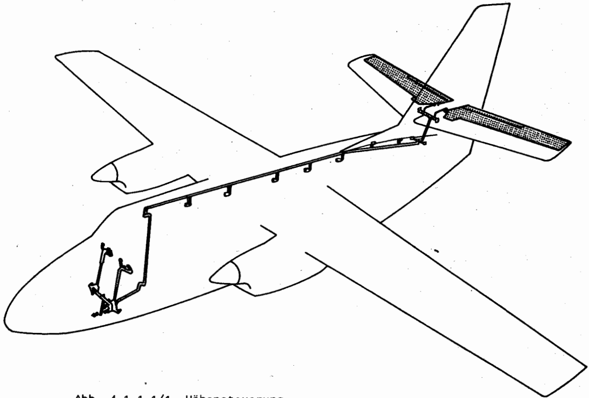
Abb. 4.1.1.1/1 Höhensteuerung
