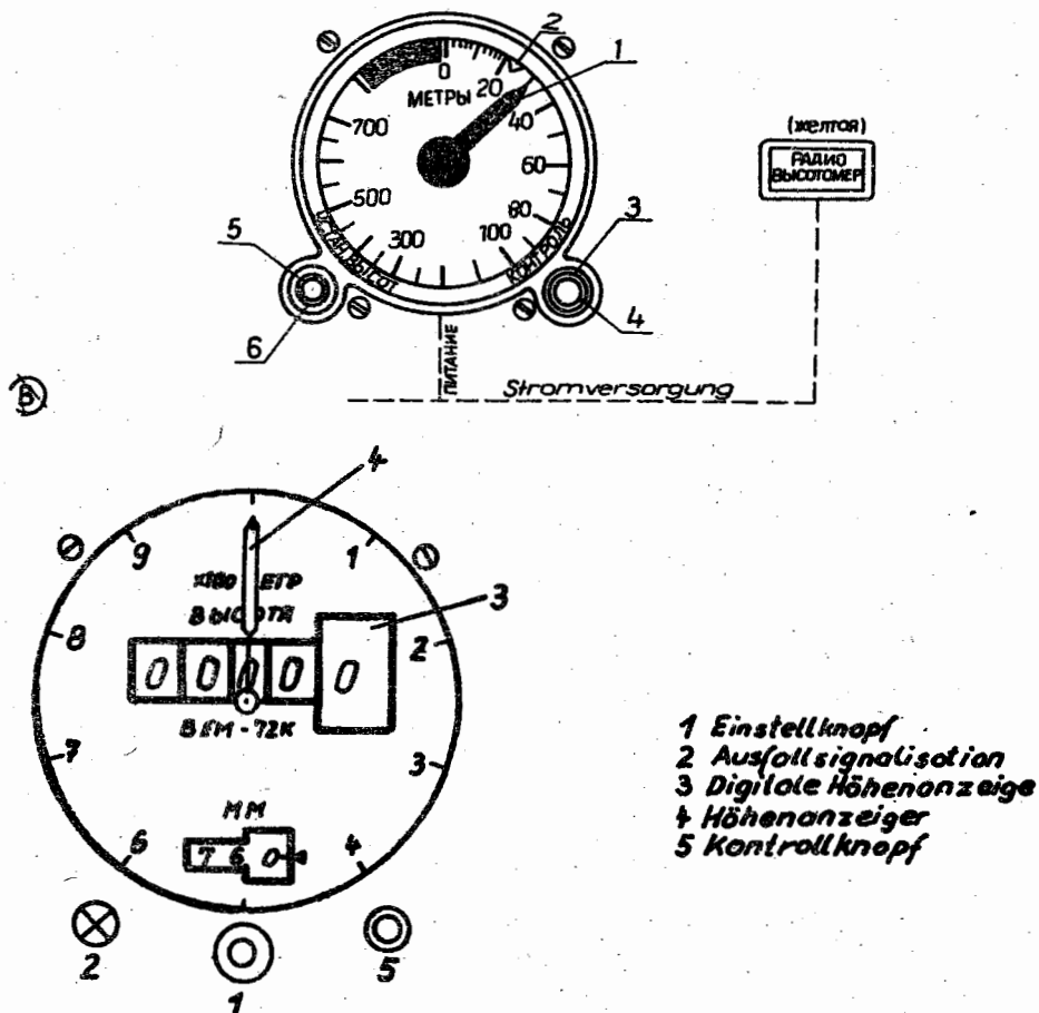
Abb. 4.1.11./3 Funkhöhenmesser und Höhenmesser БЭМ-72К
