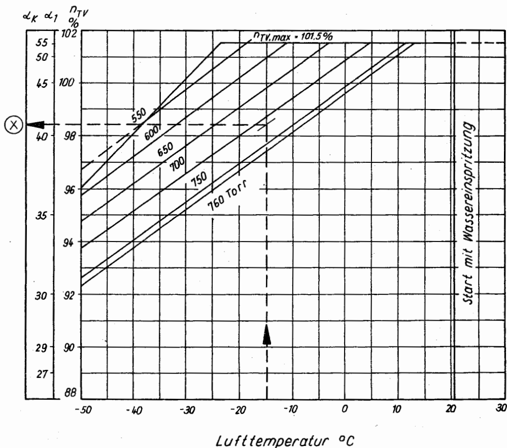
Abb. 4.1.2/3 Grafik für die Einstellung des regulierbaren Anschlages ( M 601 B ) für die max. Startleistung Gültig für n_{LS} = 2080 \text{ min}^{-1}
