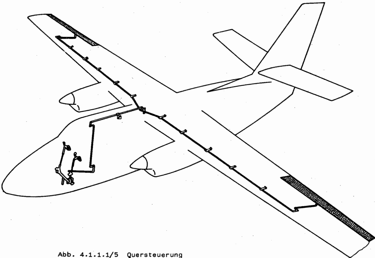
Abb. 4.1.1.1/5 Quersteuerung
