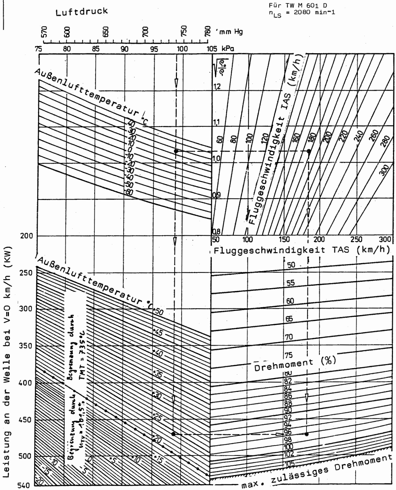
Abb. 4.1.2/4 Diagramm zur Einstellung der max. Startleistung
